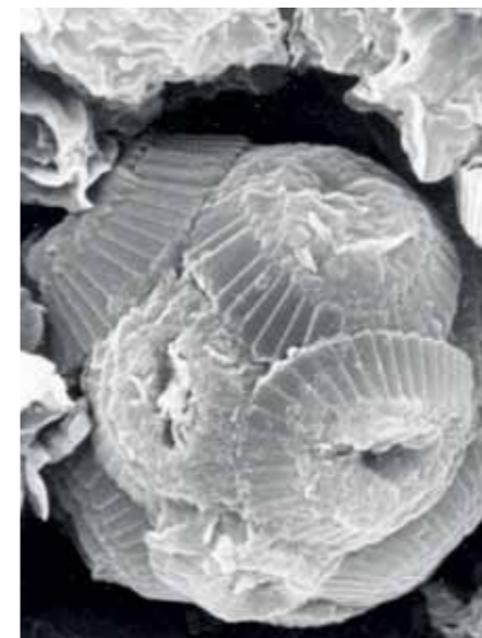
Rasterelektronenmikroskopische Aufnahme von Nannofossilien (Coccosphäre aus Anthering, Salzburg, 55 Millionen Jahre).
